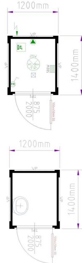
WC65FRD073235-7035.dwg
